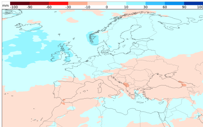
Niederschlagsentwicklung 03.03. - 10.03. (Woche 3)
