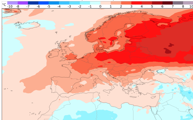
Temperaturentwicklung 03.03. - 10.03. (Woche 3)
