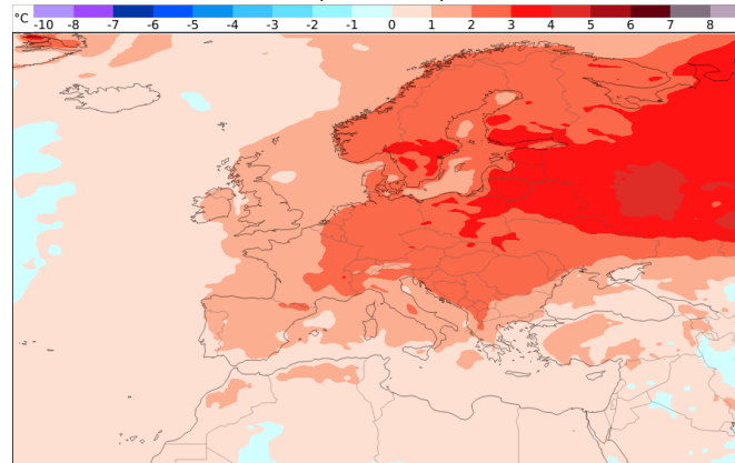
Temperaturentwicklung 10.03. - 17.03. (Woche 4)
