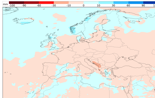
Niederschlagsentwicklung 10.03. - 17.03. (Woche 4)
