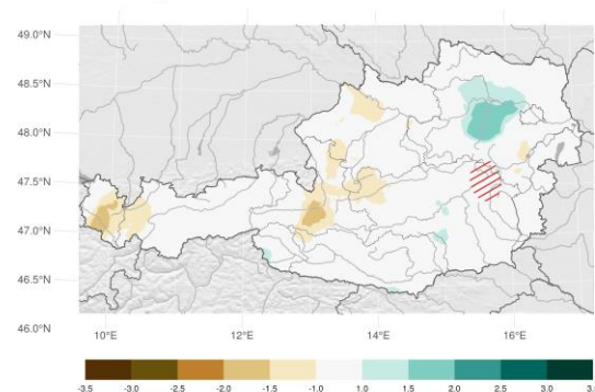
Index der klimatischen Wasserbilanz (Dürreindex) der letzten 365 Tage; Flächenmittel: -0.17
