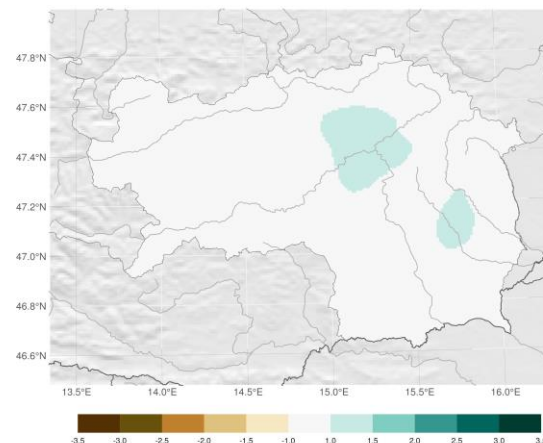
Index der klimatischen Wasserbilanz (Dürreindex) der letzten 30 Tage; Flächenmittel: 0.32
