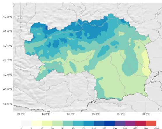
Niederschlagssumme der letzten 30 Tage Flächenmittel: 64.91 mm
