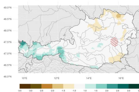
Index der klimatischen Wasserbilanz (Dürreindex) der letzten 365 Tage; Flächenmittel: 0.08
