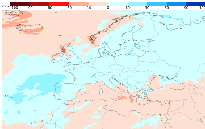
Niederschlagsentwicklung 14.10. - 21.10. (Woche 3)
