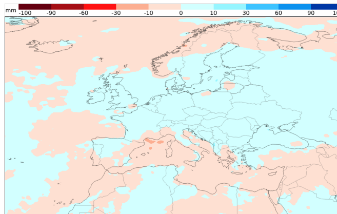
Niederschlagsentwicklung 21.10. - 28.10. (Woche 4)
