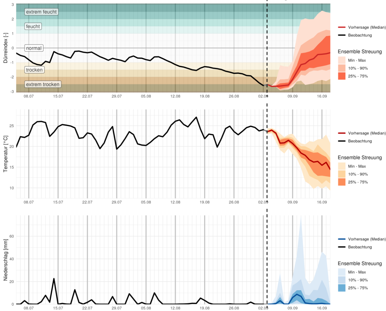
beobachtete Niederschlagssumme (60 Tage): 108.8 mm, vorhergesagte Niederschlagssumme (16 Tage): 10.1 - 174.5 mm (Median 48.3 mm)
